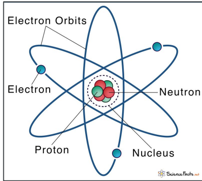
Atomo ~ 10^{-8} cm
