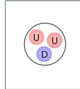
Protone ~ 10^{-13} cm ~ 10^{-24} g
