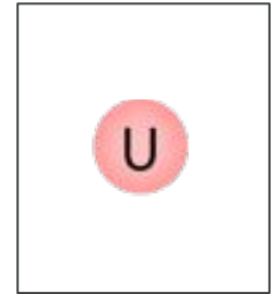
Quark ~ 10^{-16} cm
