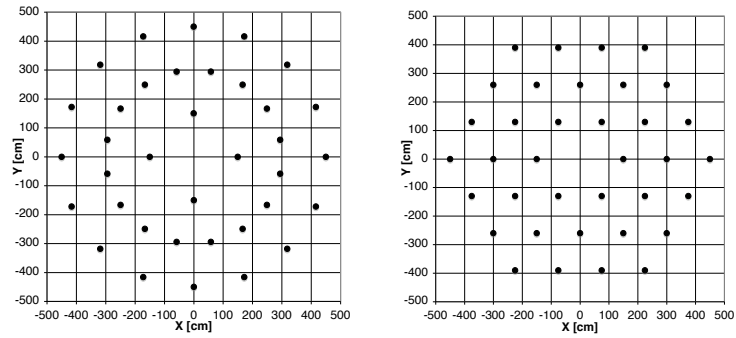
(d) Bottom / Top Array Model 4 with 36 PMTs.
