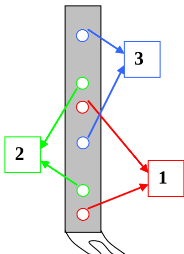
Figura 36: Posizioni per inserire i fermacavi sulle staffette di alluminio. Il fermacavo va messo con l'apertura rivolta verso il superlayer PHI 2.
