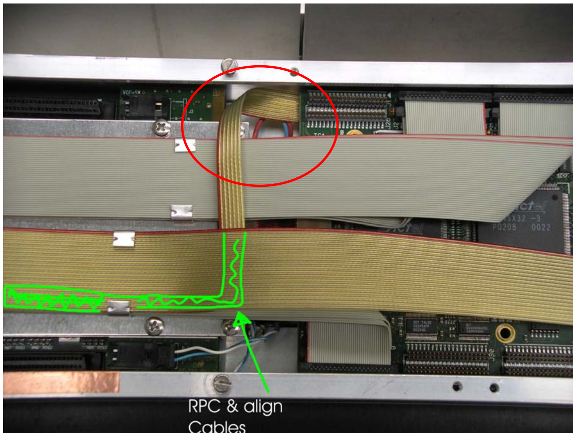
Figura 6: Cables routing in uscita dalla SB. Dettaglio su cavi RPC e Allineamento.
