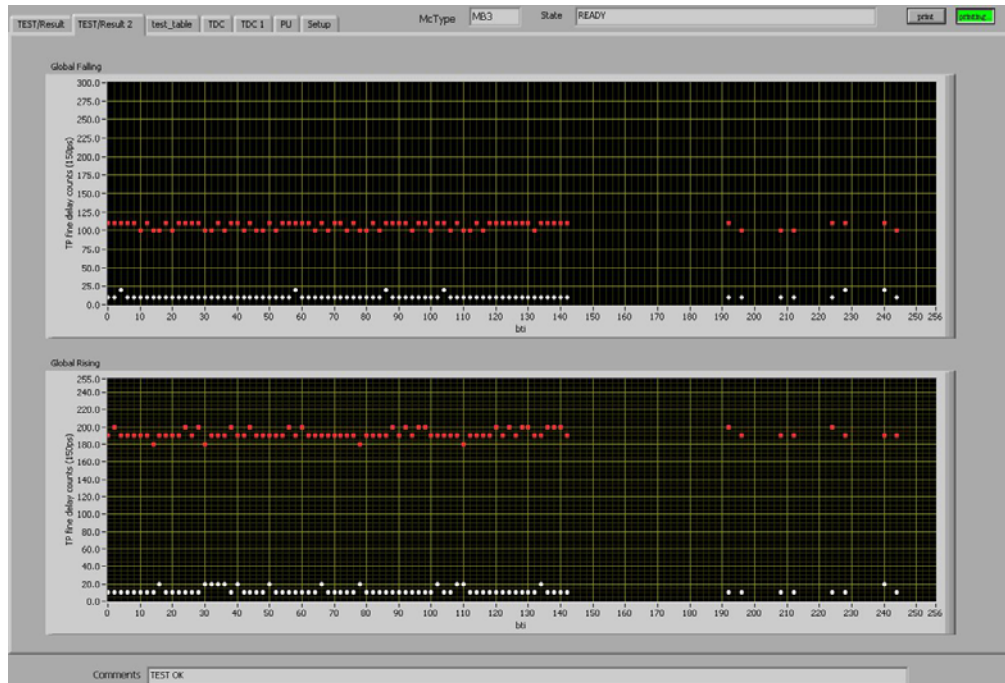
Figura 35: Output del Test di BTI skew: I due grafici mostrano in ascissa il BTI impulsato col test pulse e in ordinata il valore di delay sulla fase del test pulse in cui gli errori vanno a 0 (global falling plot) e quello in cui aumentano (global rising plot). Lo sfasamento in ordinata di tutti i punti deve essere compreso in un intervallo tipico di 3-4 ns.
