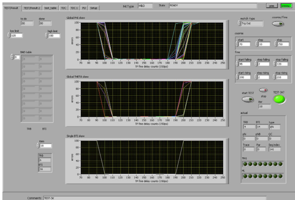
Figura 34: Output del test di Bti Skew: ogni curva si riferisce agli errori (su 100 pattern per punto) eseguendo un test pulse variando la fase del segnale impulsato su un BTI. Come si vede dai primi due grafici dall'alto ci deve essere una regione in cui il numero di errori e' inferiore a 10 (tra 120 e 180) e le due zone in cui iniziano gli errori devono essere sovrapposte per tutti i BTI con uno sfasamento di 3-4 ns (ricorda : 1 tick nell'asse x = 150 ps). L'ultimo grafico permette di visualizzare la curva singolarmente per ciascun BTI.
