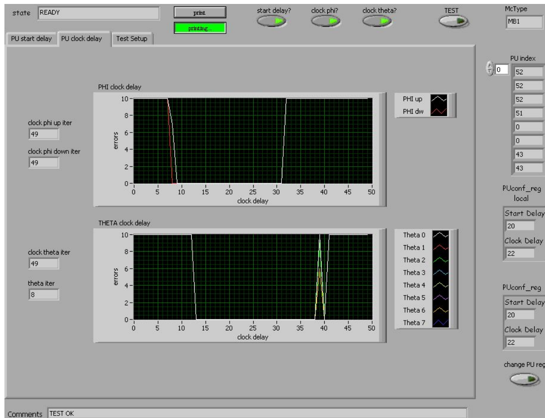
Figura 25: Pattern Unit Calibration per un minicrate MB1
