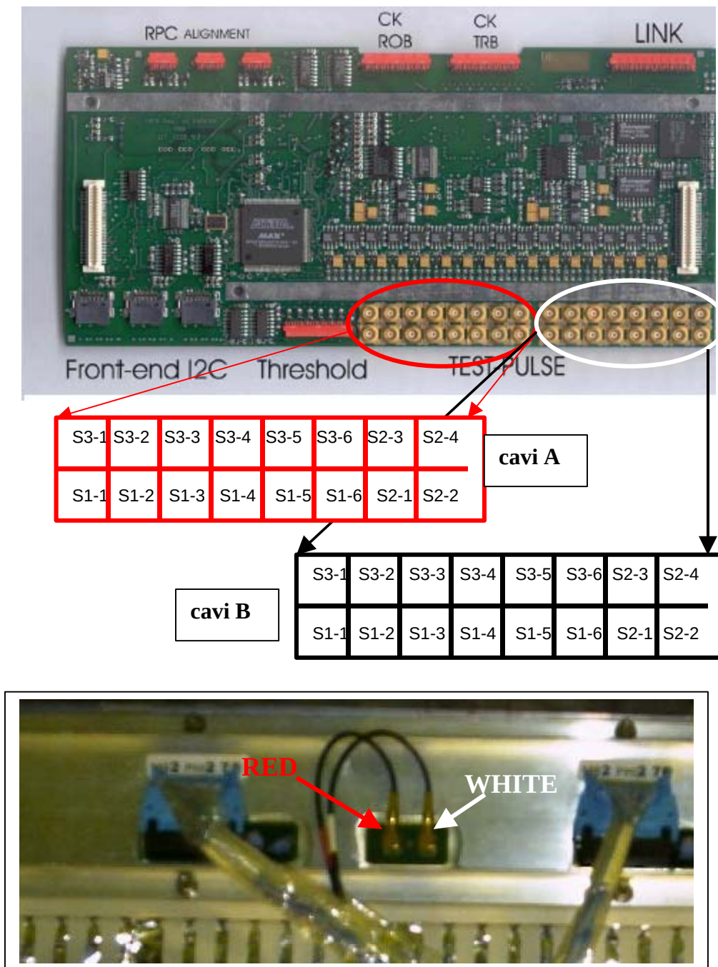
Figura 32: connessione dei cavi test-pulse
