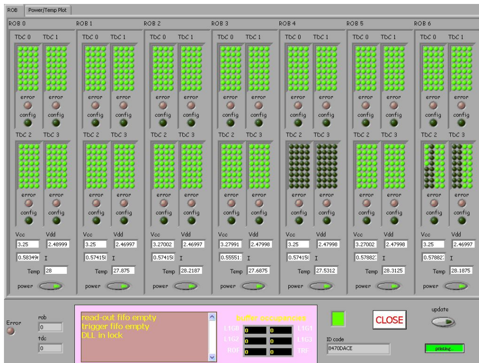
Figura 24: TDC status per MB3
