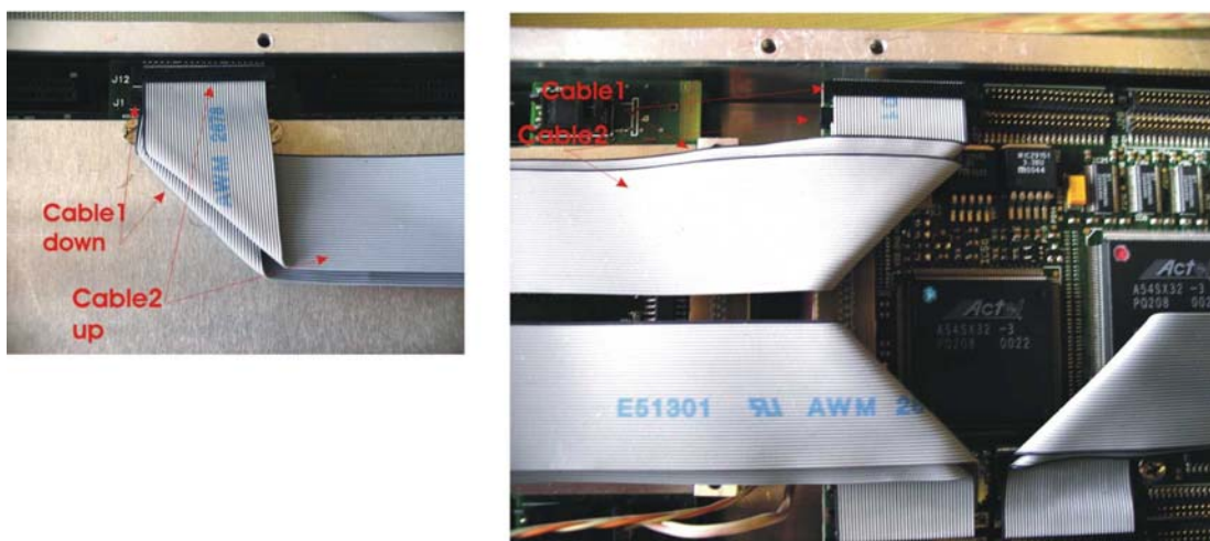
Figura 13: Connessioni e disposizione dei cavi di trigger: particolare.
