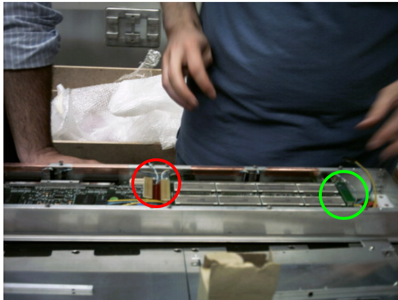
Figura 2: Inserimento TRB; si noti l'End Trigger Bus (verde) e il Trigger Bus (rosso).
