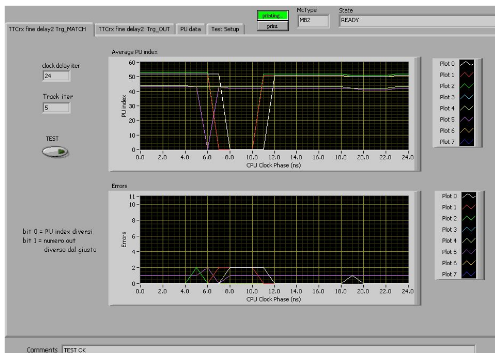
Figura 31: Esempio di output del Test Serializers per un MB2: Si noti come la TRB5 (la THETA 1 per un MB2) abbia sempre errori su tutto l'intervallo dello scan di fase. Questo indica un malfunzionamento della scheda o un difetto nella connessione di essa alla Server Board indipendente dalla sincronizzazione reciproca.
