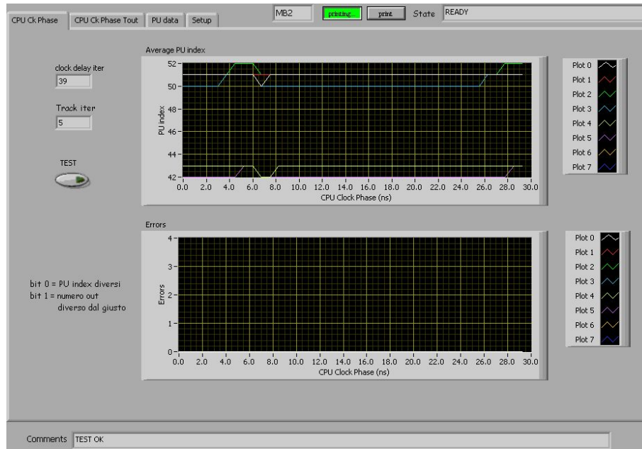
Figura 28: Esempio di output corretto per il test CPU CK Phase (MB2): il primo grafico in alto mostra in quale time-slot della Pattern Unit (PU index) il dato e' trovato correttamente in funzione della fase del clock alla CPU che induce lo start dell'emulazione dei BTI . Ciascun Plot nella legenda si riferisce ad una diversa TRB. Si noti: lo sfasamento di 7 time-slot tra le board PHI e quelle THETA; una regione di circa 4 ns in cui la time-slot non e' stabile. Questa ultima osservazione indica che la fase del clock alla CPU non assicura che le tracce siano emulate dai dispositivi con un timing stabile e che siano quindi attese in uscita alla stessa time-slot. Per ciascun punto vengono emulate 10 tracce. Nel secondo grafico sono mostrati gli errori secondo il codice nella legenda a sinistra. Possono esserci errori tipicamente nella zona in cui il clock e' critico. Si osservi come per un valore di 12 ns il clock e' in una regione stabile.
