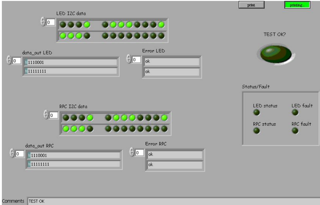
Figura 22: Output Corretto per il test Led-RPC
