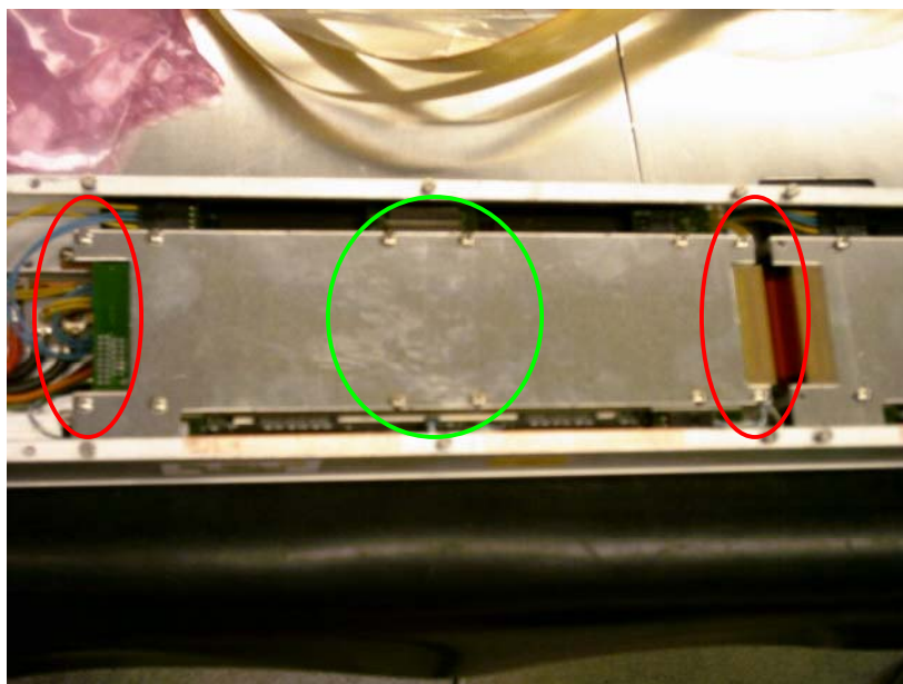
Figura 10: Viti per il fissaggio dei coperchi di dissipazione delle TRB.
