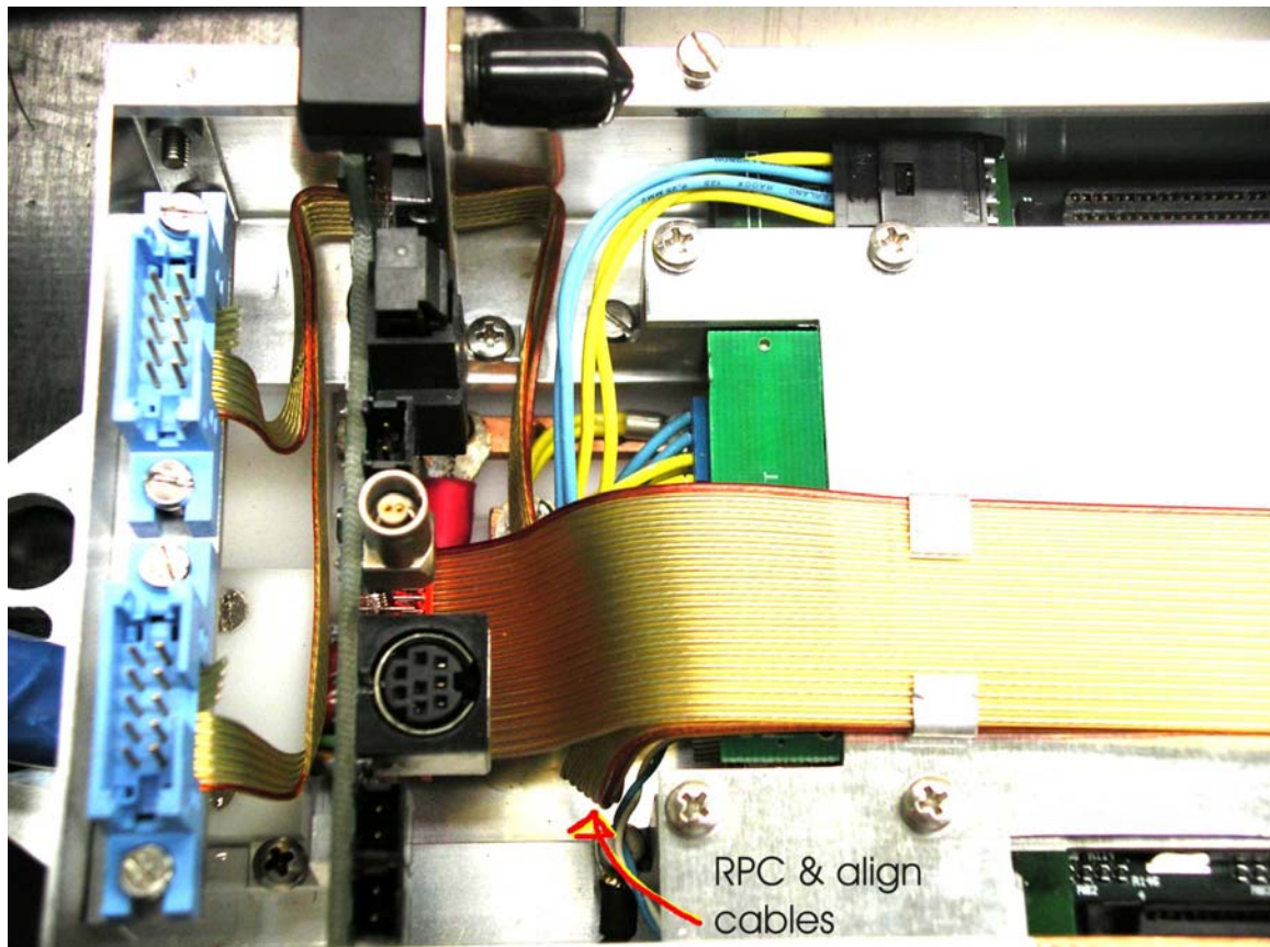
Figura 14: Connettore RPC-Allineamento e routing dei cavi attorno alla Link Board.
