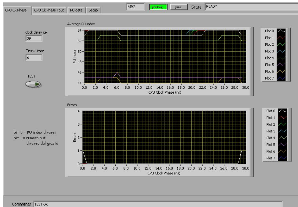
Figura 29: Esempio di corretto output per il Test CPU CK Phase (MB3)
