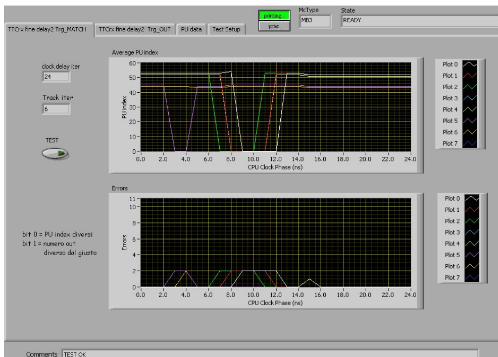
Figura 30: Output del Test Serializers per un MB3. Si osservi come un valore della fase di clock uguale a 0 (il default) sia accettabile. L'interpretazione dei plot e' simile a quelli in Figura 28. Ogni plot si riferisce ad una diversa TRB, mentre la fase del clock e' quella alla Server Board.
